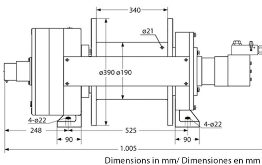
Dimensions in mm/ Dimensiones en mm
